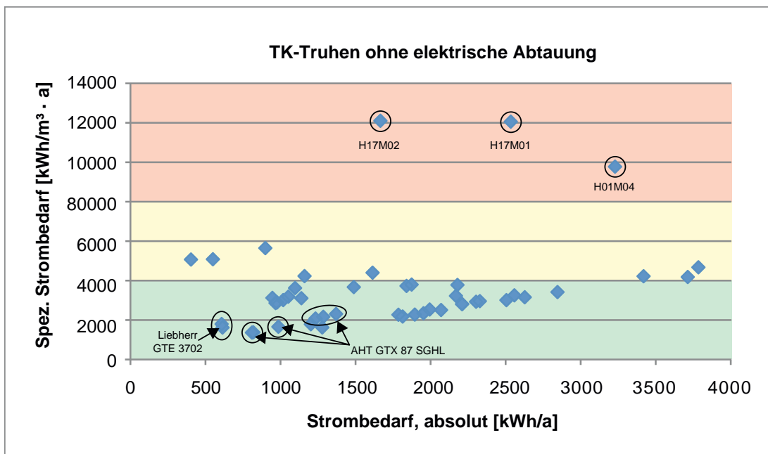
Abb. 22. Strombedarf TK-Truhen ohne elektrische Abtaung
