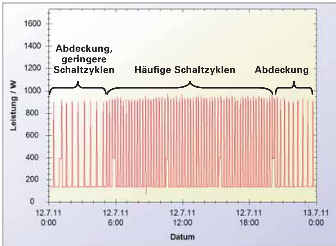
Abb. 40. Wirkung der Nachtdeckung
