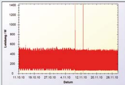
Abb. 14. Lastgang Periode, H02M01
