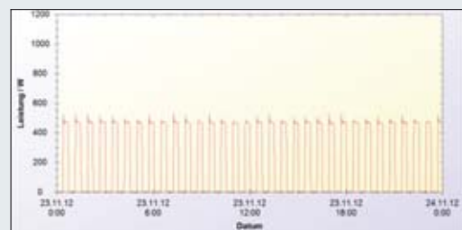
Abb. 101. Lastgang Tag, AHT
