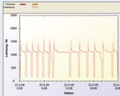
Abb. 140. Lastgang Tag, H09M09
