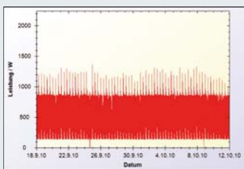
Abb. 60. Lastgang Periode, H12M01
