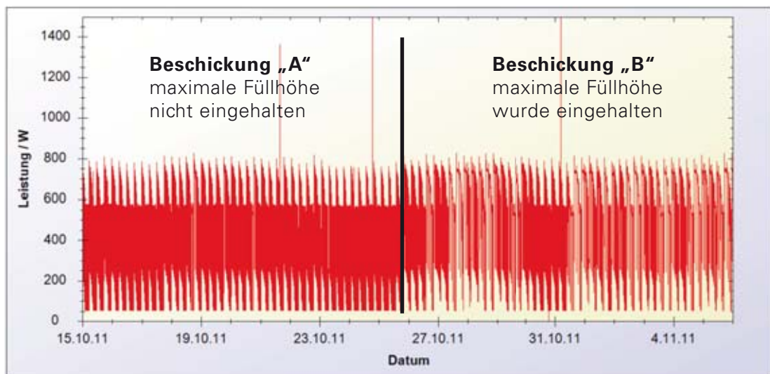
Abb. 44. Lastgang Periode, Füllhöhenwechsel
