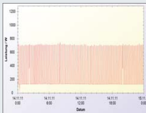
Abb. 30. Lastgang Tag, H09M01
