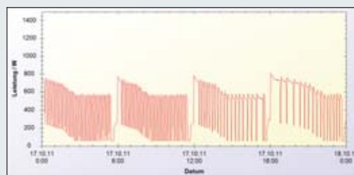
Abb. 65. Lastgang Tag, H13M01
