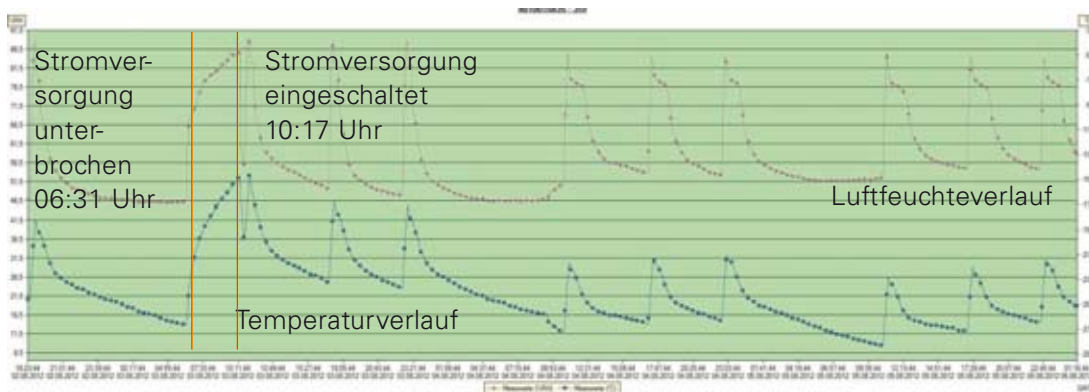
Abb. 66. Temp.- rel.-Luftfeuchteverlauf bei der H09M04-TK-Truhe
