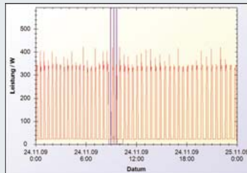
Abb. 21. Lastgang Tag, AHT Wien
