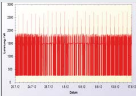
Abb. 131. Lastgang Periode, H09M04
