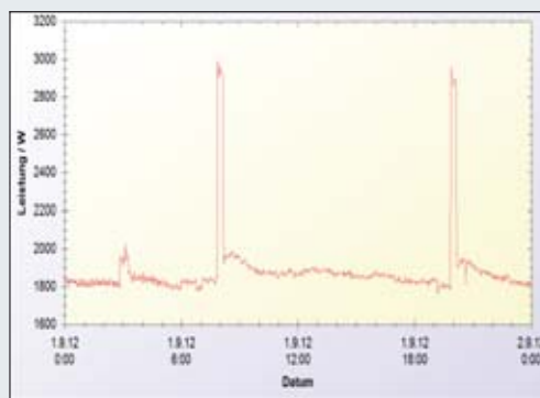
Abb. 75. Lastgang Tag, H07M07
