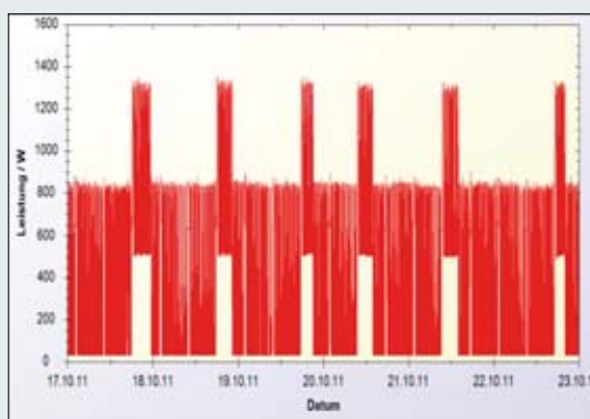
Abb. 48. Lastgang Woche, H08M02
