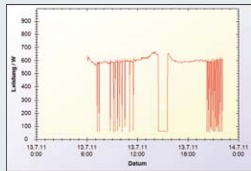
Abb. 42. Lastgang Tag, H09M02
