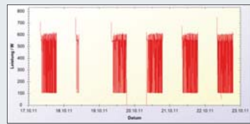
Abb. 27. Lastgang Woche, H05M03
