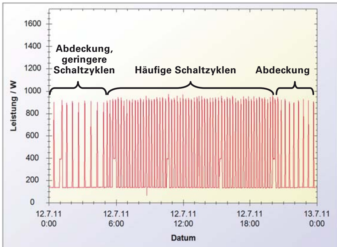
Abb. 40. Wirkung der Nachtabdeckung
