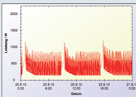
Abb. 61. Lastgang Tag, H12M01
