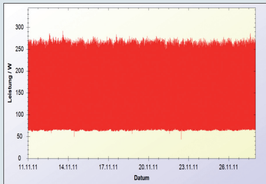
Abb. 8. Lastgang Periode, Megacooler
