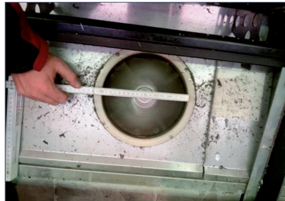
Abbildung 35. Einbau im Kühlmöbel 80
