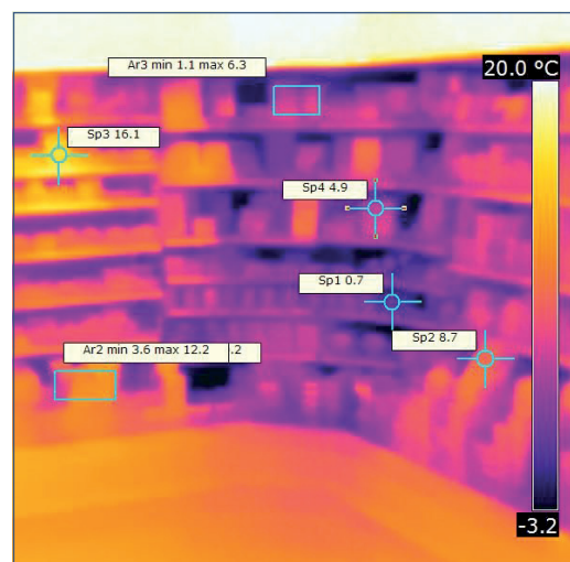
Abbildung 12. Wärmebild Eck-Kühlregal
