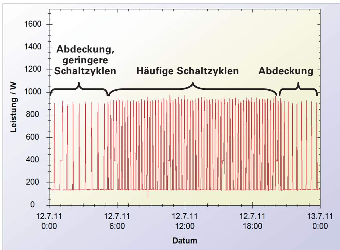
Abb. 40. Wirkung der Nachtabdeckung
