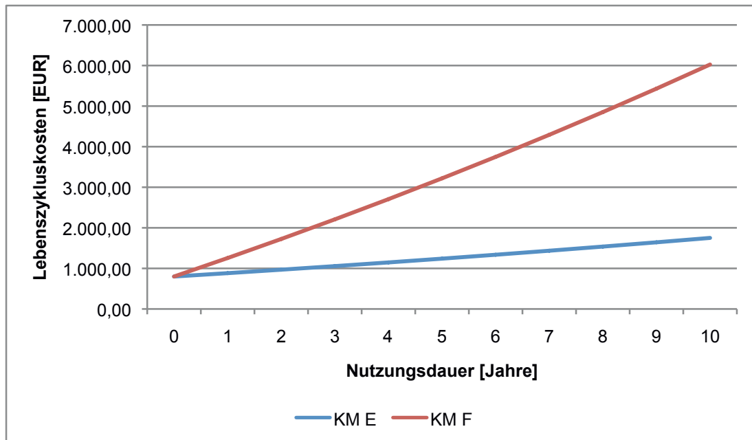
Abb. 32. Lebenszykluskosten TK-Truhen, geschlossen
