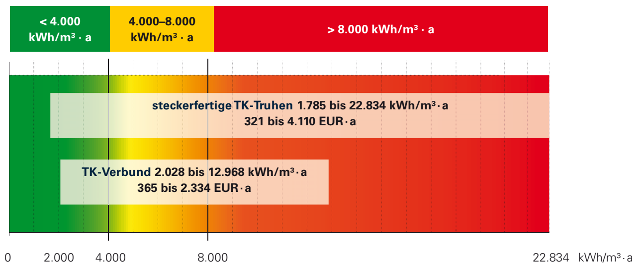
Abb. 70. Strombedarf TK-Truhen
