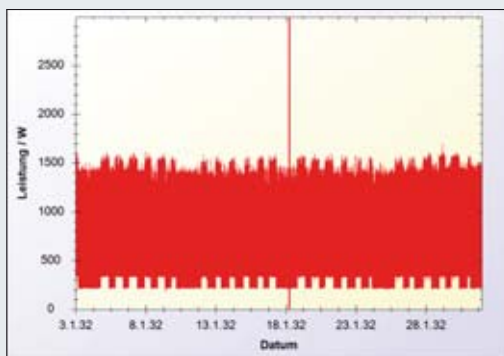
Abb. 70. Lastgang Periode, H18M01
