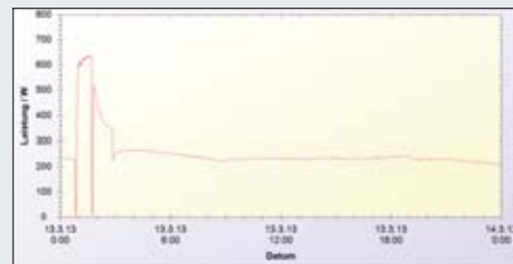
Abb. 126. Lastgang Tag, AHT Athen 210
