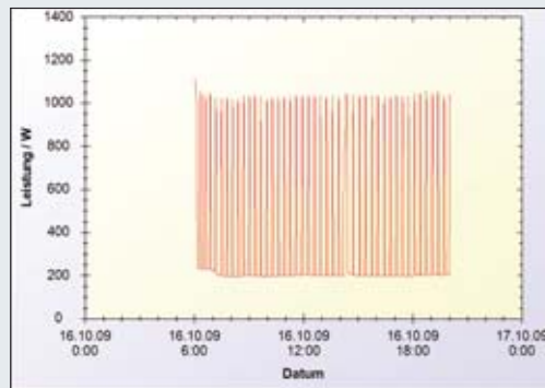
Abb. 52. Lastgang Tag, H08M03
