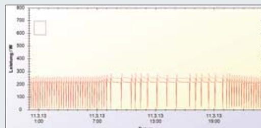
Abb.130. Lastgang Tag, AHT
