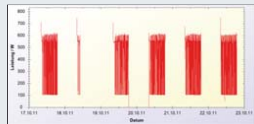
Abb. 27. Lastgang Woche, H05M03
