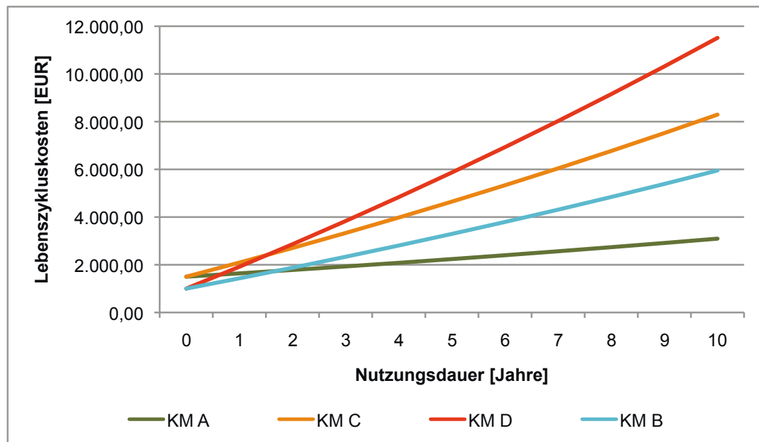
Abb. 29. Lebenszykluskosten Getränkeregale, geschlossen
