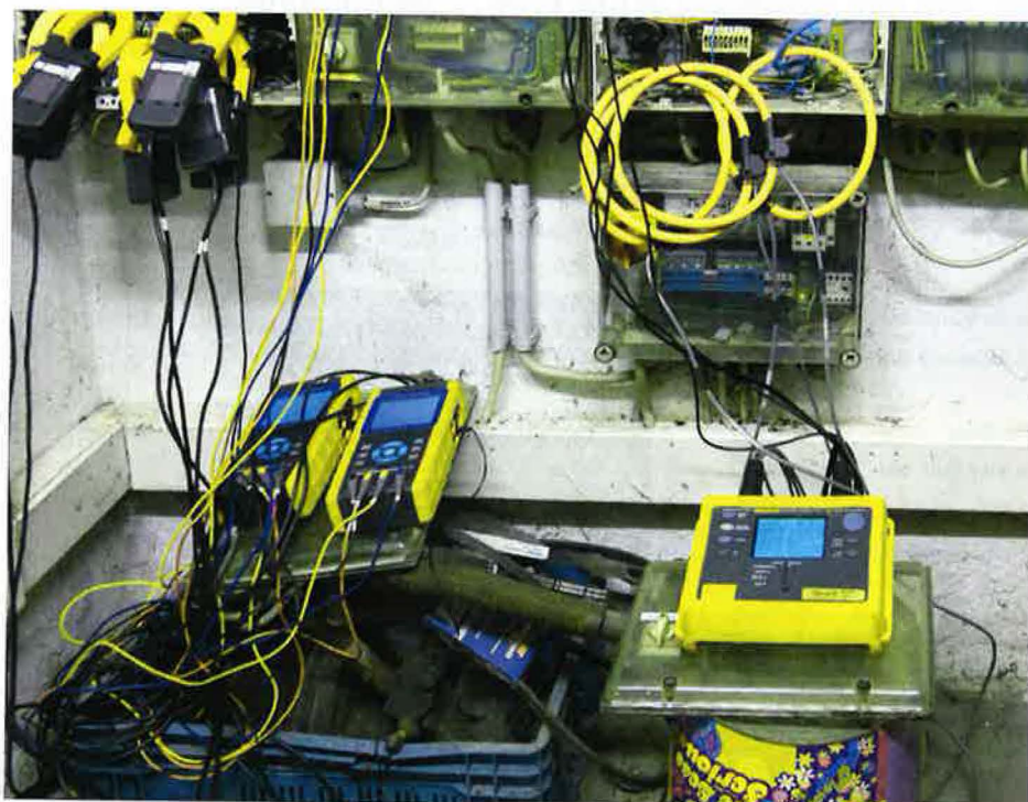
Typischer Messaufbau in älteren Unterverteilungen
